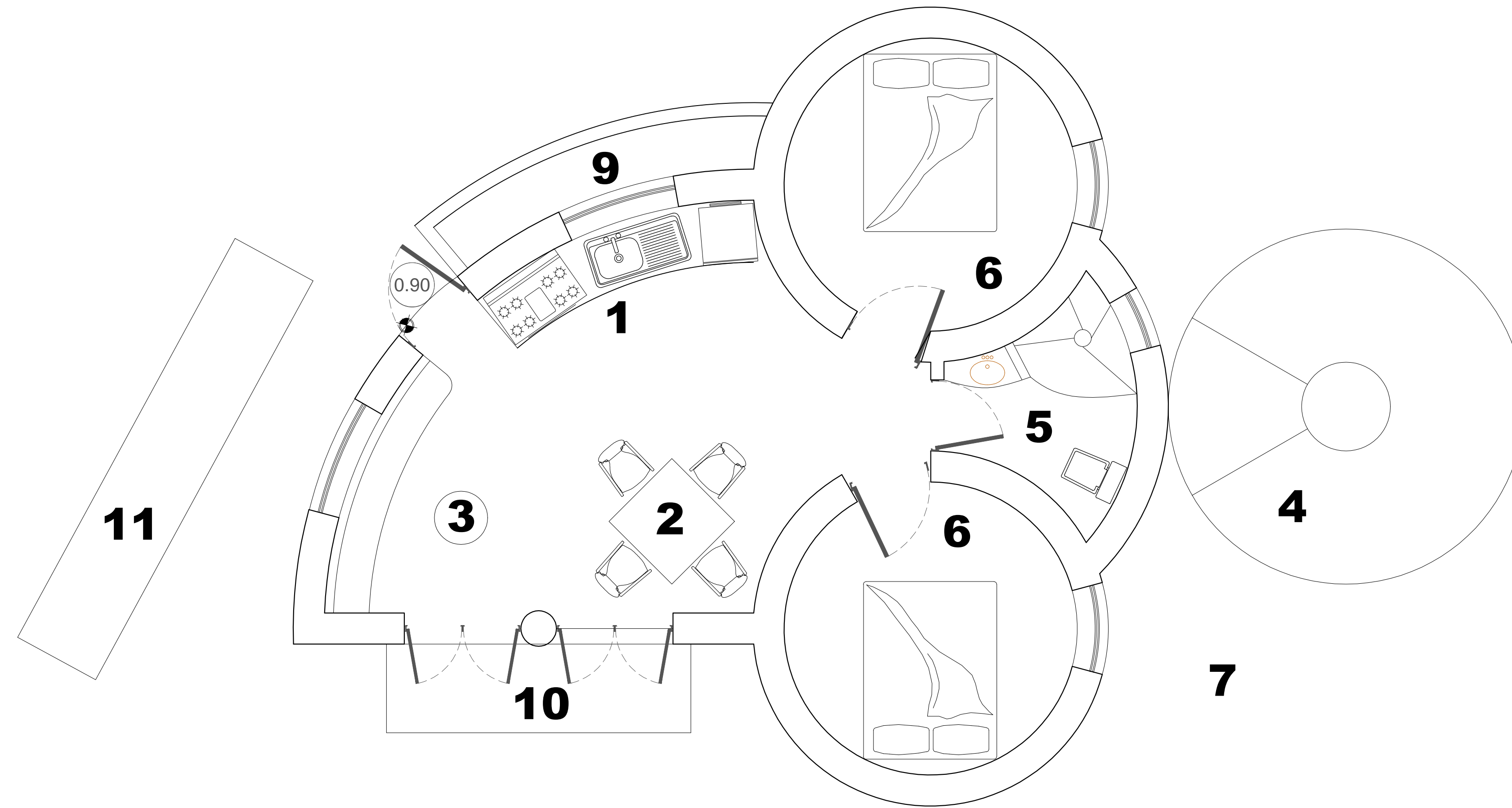
PLANTA ARQUITECTÓNICA
