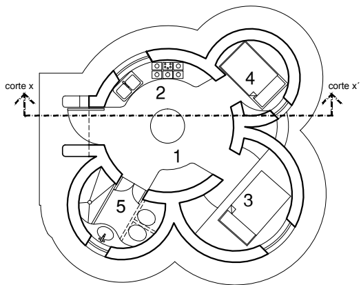
PLANTA ARQUITECTÓNICA
