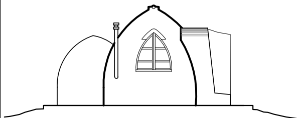
FACHADA LONGITUDINAL
